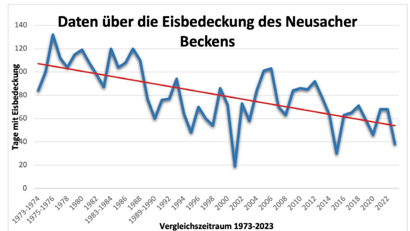
Diagramm 2: Eisbedeckung des Ostteils in Tagen im Vergleichszeitraum 1973-2023 (Quelle: Norbert Jank)
