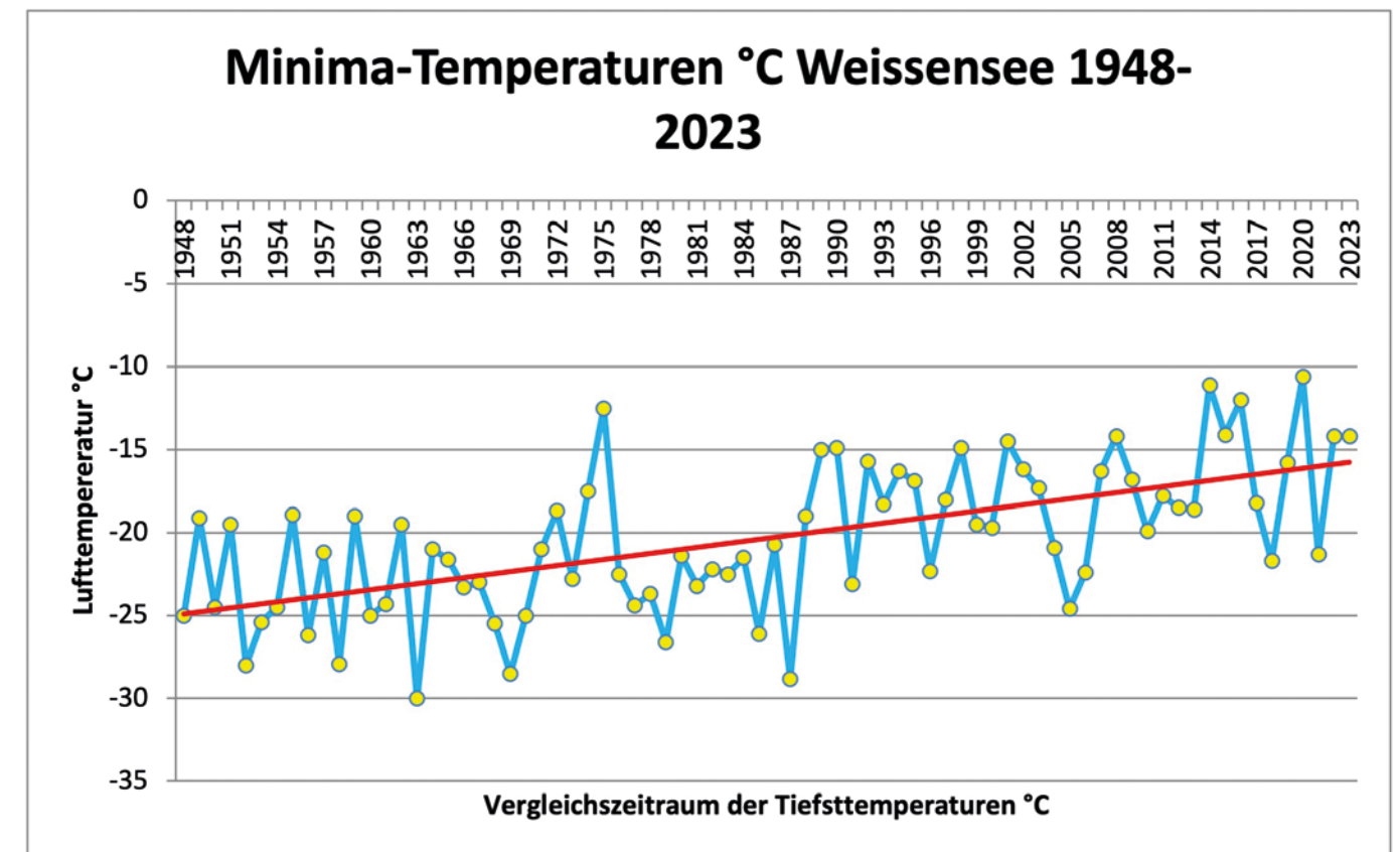
Diagramm 1: Trendlinie – Minima-Temperaturen in °C im Vergleichszeitraum 1948-2023 – Quelle: GeoSphere Austria
